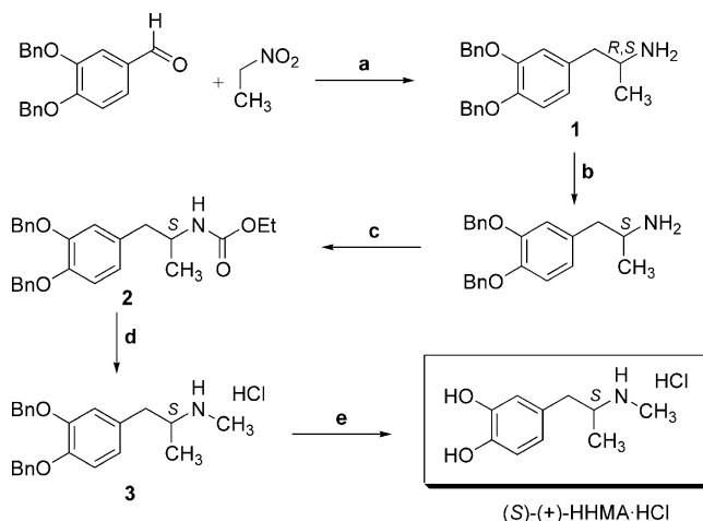
Scheme 1. Synthesis of enantiomerically enriched (S)-HHMA·HCl. a: 1) \text{CH}_3\text{CO}_2\text{NH}_4 ; 2) \text{LiAlH}_4 ; b: resolution; c: \text{ClCO}_2\text{Et} ; d: 1) \text{LiAlH}_4 ; 2) \text{HCl} ; e: \text{H}_2 , Pd-C, MeOH.
